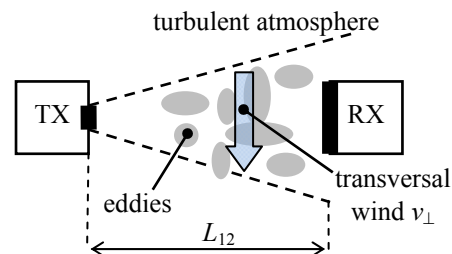
Fig. 1 FSO link.
